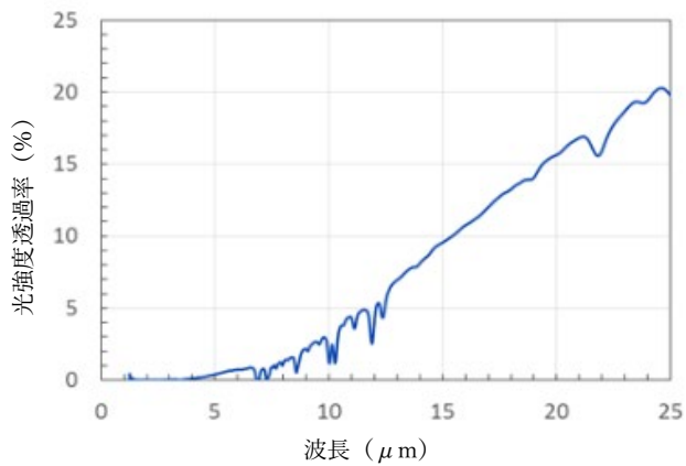
BPP フィルムの透過特性 (FT-IR による測定値)
