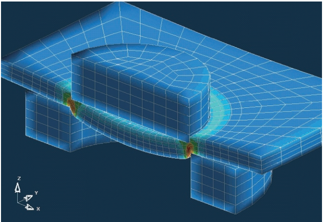
応力解析による超硬合金精密金型の設計。高度な金型設計により加工品質を向上。
