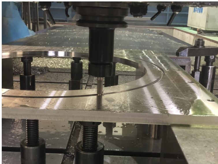
ステンレスプレート アリ溝加工
