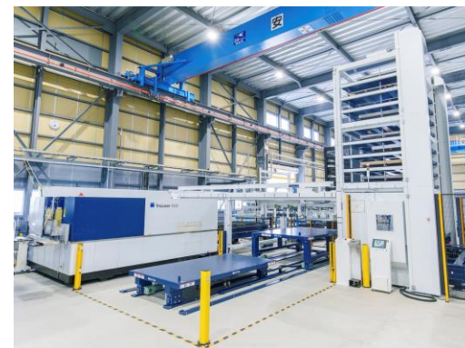
レーザーと連結した 自動搬送システム
