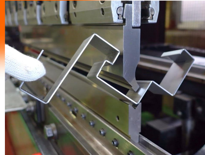
ベンダーによる曲げ加工
