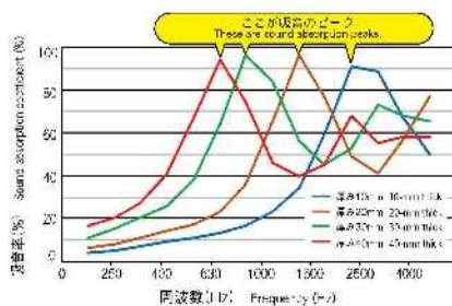
吸音率 (垂直入射法) オプセル LC-300#1 Sound absorption coefficient (normal incidence) of OPCELL LC-300#1
