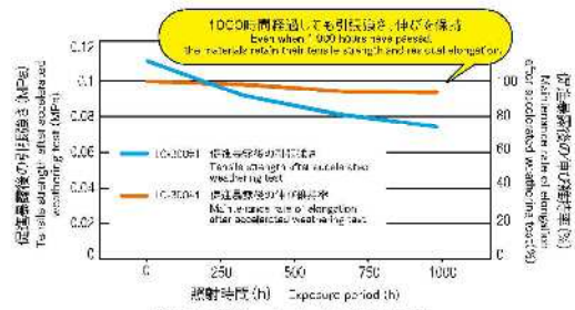
耐候性試験 オプセル LC-300#1 (サンシャインウェザーメーターによる促進曝露試験)
